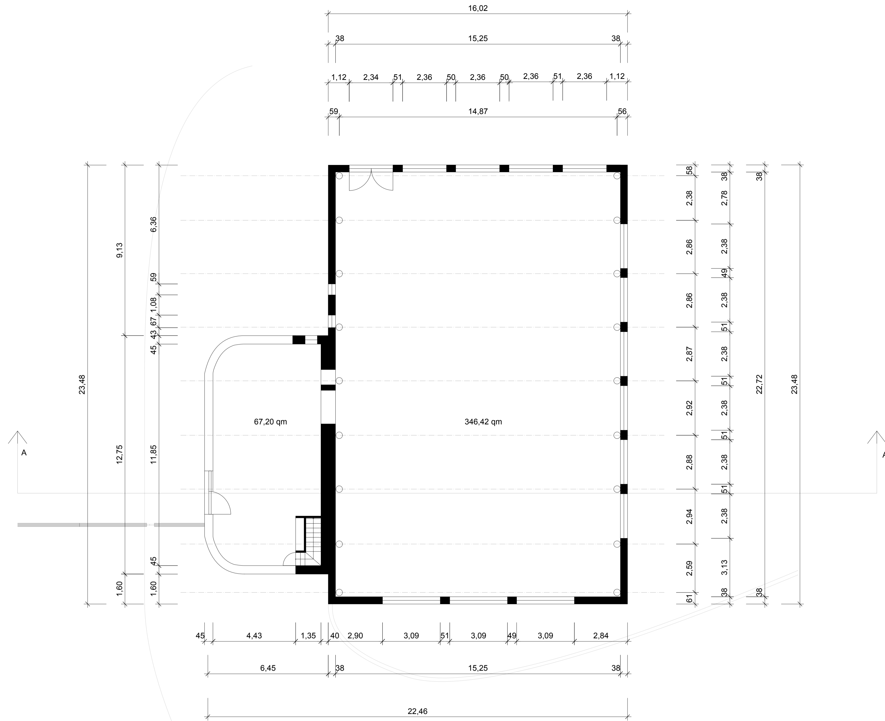
Grundriss Pforte Ost und Gebäude 48(2) M 1:100
